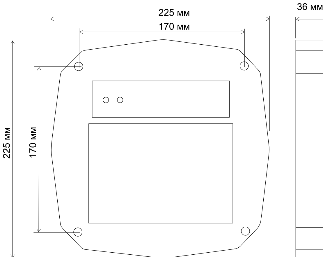
Рис.1 Габаритные размеры.
